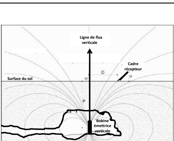
Figure 5 : ARCANA : principe, coupe verticale
