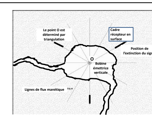
Figure 6 : ARCANA: principe, coupe horizontale
